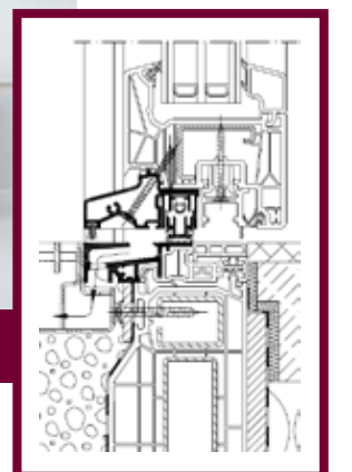
0 mm Schwelle
