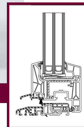
20 mm Schwelle
