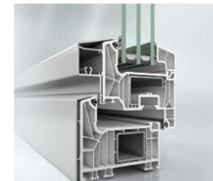
TopAlu Pure
