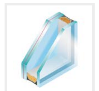
P4A Sicherheitsglas
